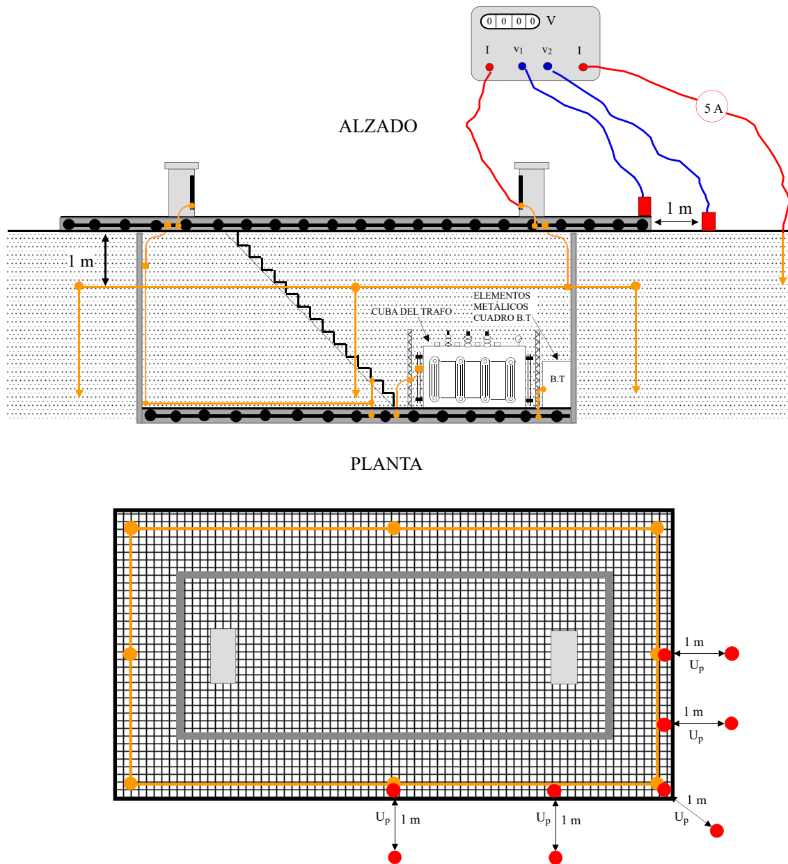
Figura 26.- Medida de la tensión de paso, U_{pam2} , con un pie en la acera y otro en el terreno del CTPS.
