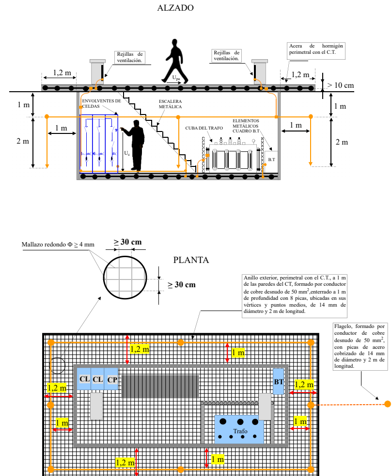
Figura 5.- Electrodo de puesta a tierra del CTPS
