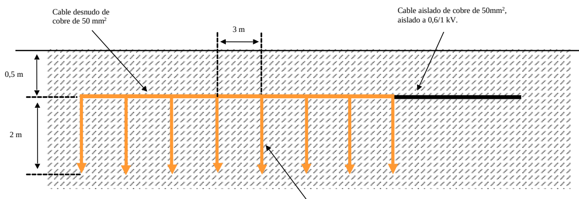
Figura 9.- Configuración CPT – CTL – 8P2, ( U_n = 30 kV) el CTOU
