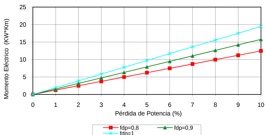
Gráfico pérdidas de potencia U=400V XZ1-Al Sec. 50 mm 2
