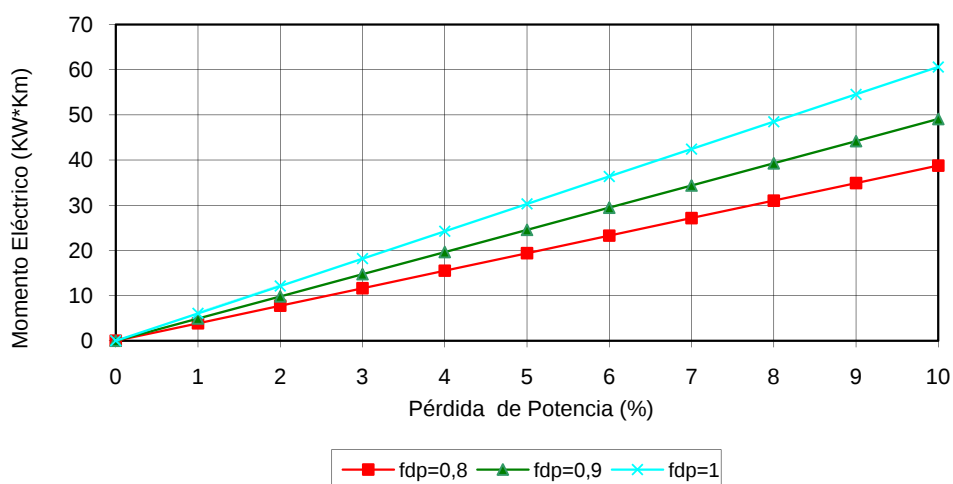
Gráfico pérdidas de potencia U=400V XZ1-Al Sec. 150 mm 2
