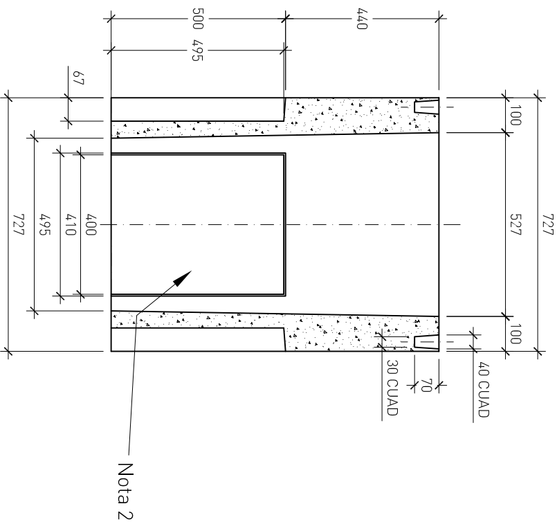
SECCION B-B
