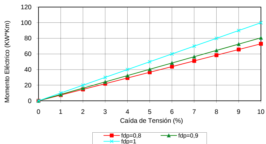
Gráfico caída de Tensión U=400V XZ1-Al Sec. 240 mm 2
