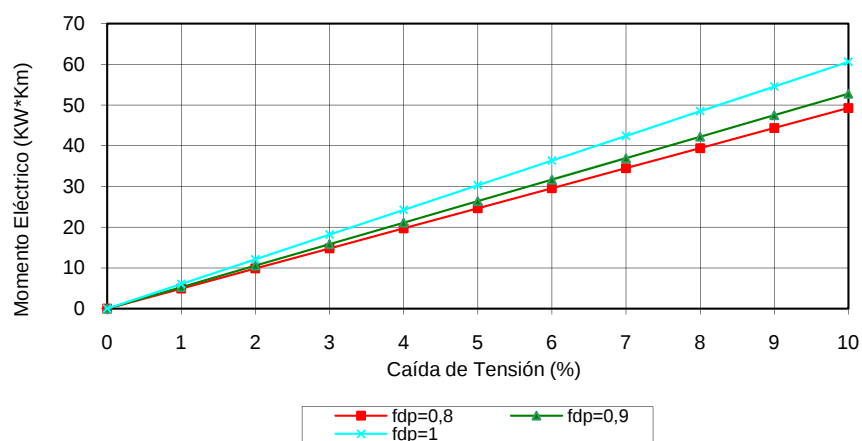
Gráfico caída de Tensión U=400V XZ1-Al Sec. 150 mm 2
