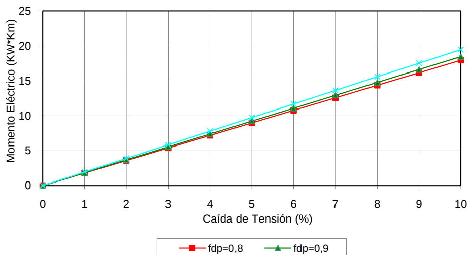
Gráfico caída de Tensión U=400V XZ1-Al Sec. 50 mm 2
