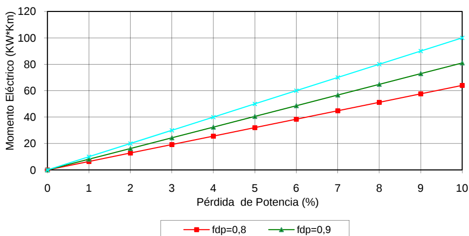
Gráfico pérdidas de potencia U=400V XZ1-Al Sec. 240 mm 2
