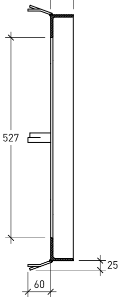
SECCION B-B'
