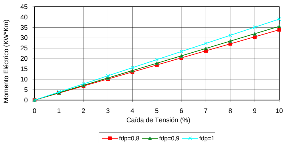
Gráfico caída de Tensión U=400V XZ1-Al Sec. 95 mm 2
