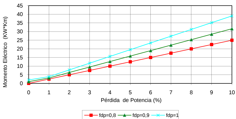
Gráfico pérdidas de potencia U=400V XZ1-Al Sec. 95 mm 2
