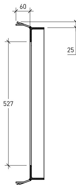
SECCION B-B'
